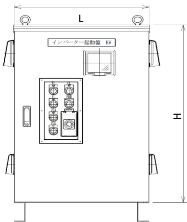
外形図
